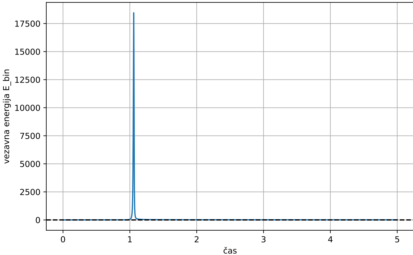
Vezavna energija dvozvezdja skozi čas ( a=2.0 , b=20 )
