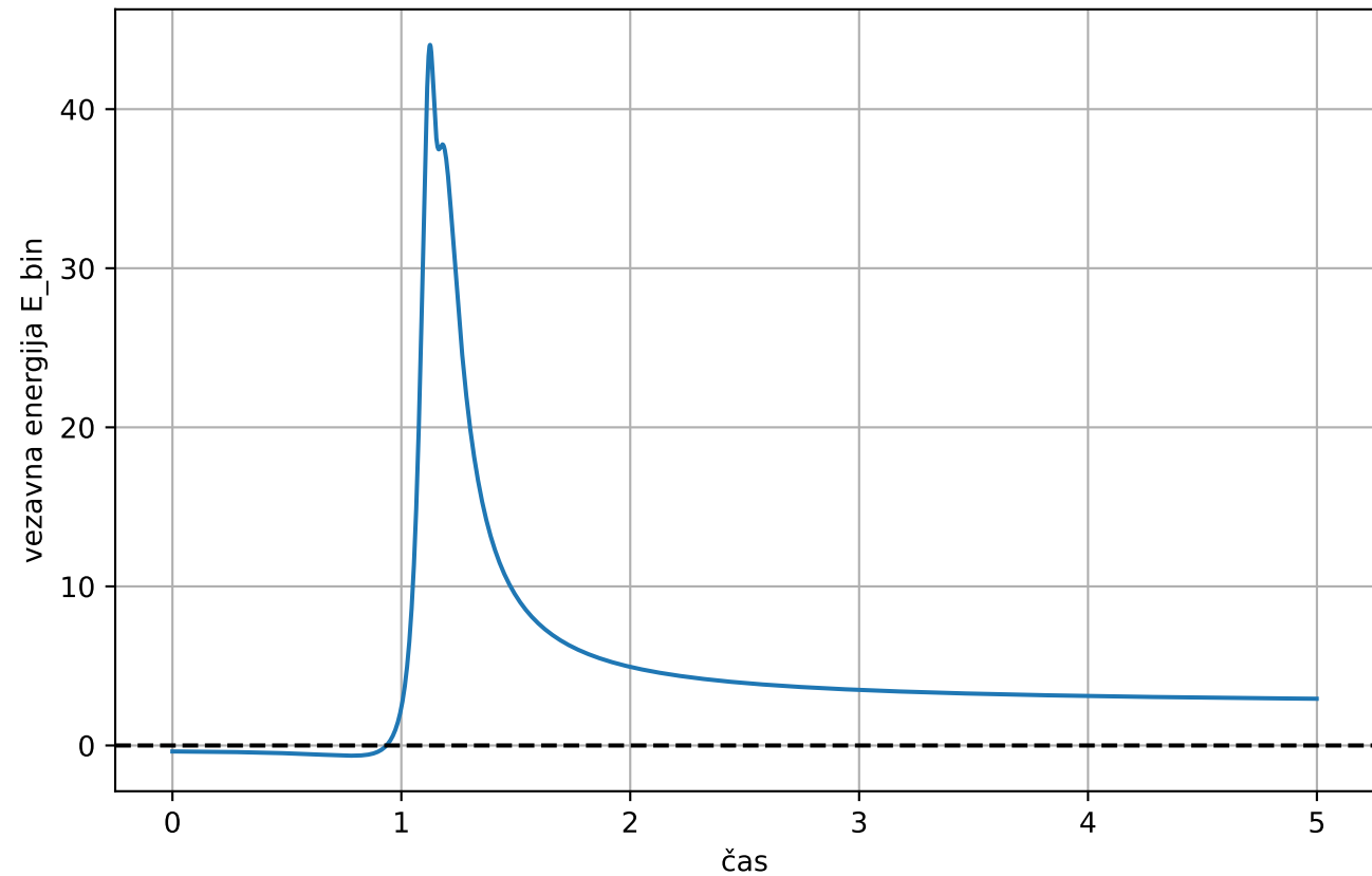
Vezavna energija dvozvezdja skozi čas ( a=2.0 , b=40 )
