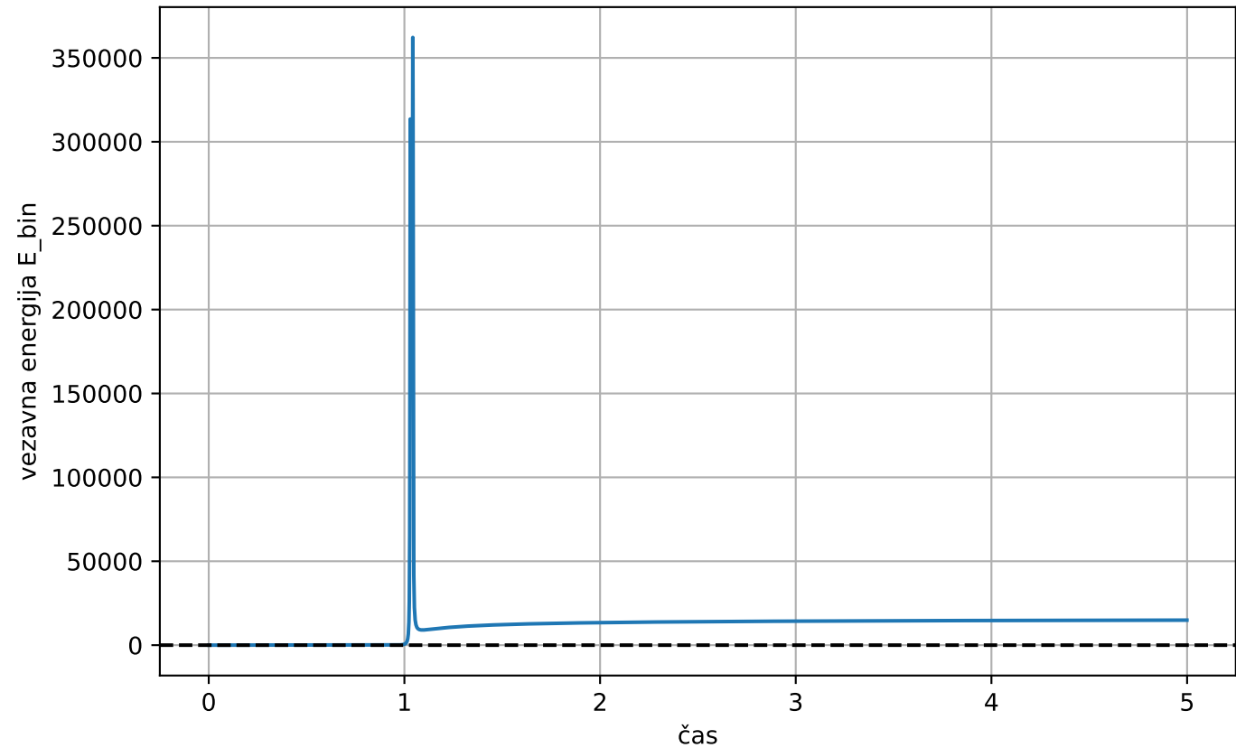
Vezavna energija dvozvezdja skozi čas ( a=3.0 , b=10 )
