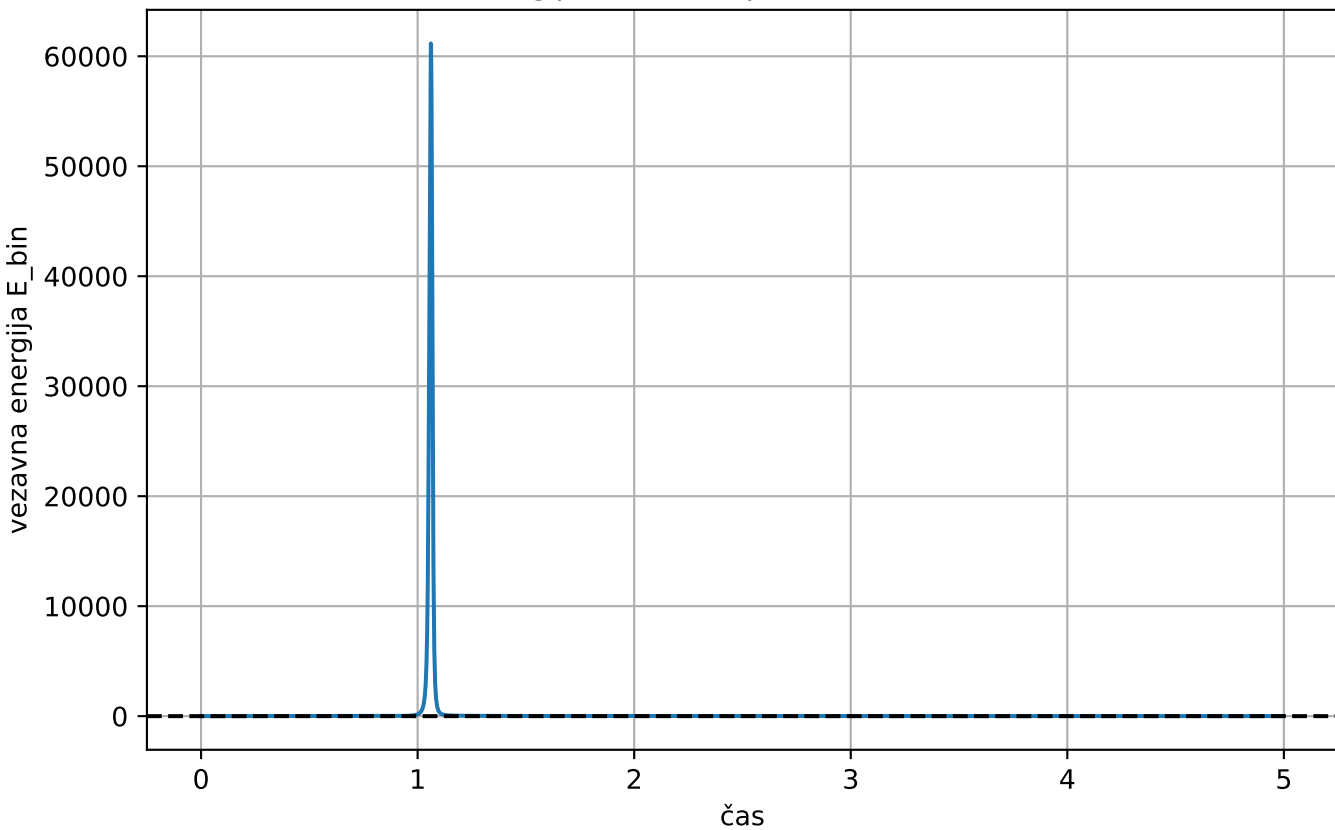
Vezavna energija dvozvezdja skozi čas ( a=3.0 , b=20 )
