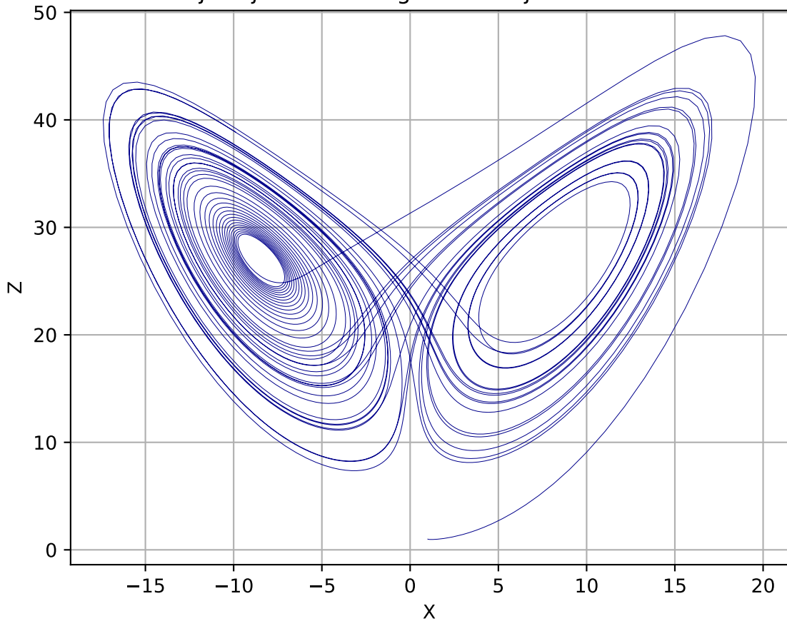
Projekcija Lorenzovega atraktorja: X-Z ravnina
