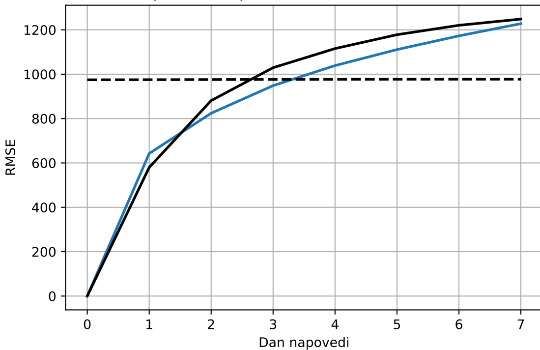
Uspešnost napovedi Z500 - Act. func. = elu
