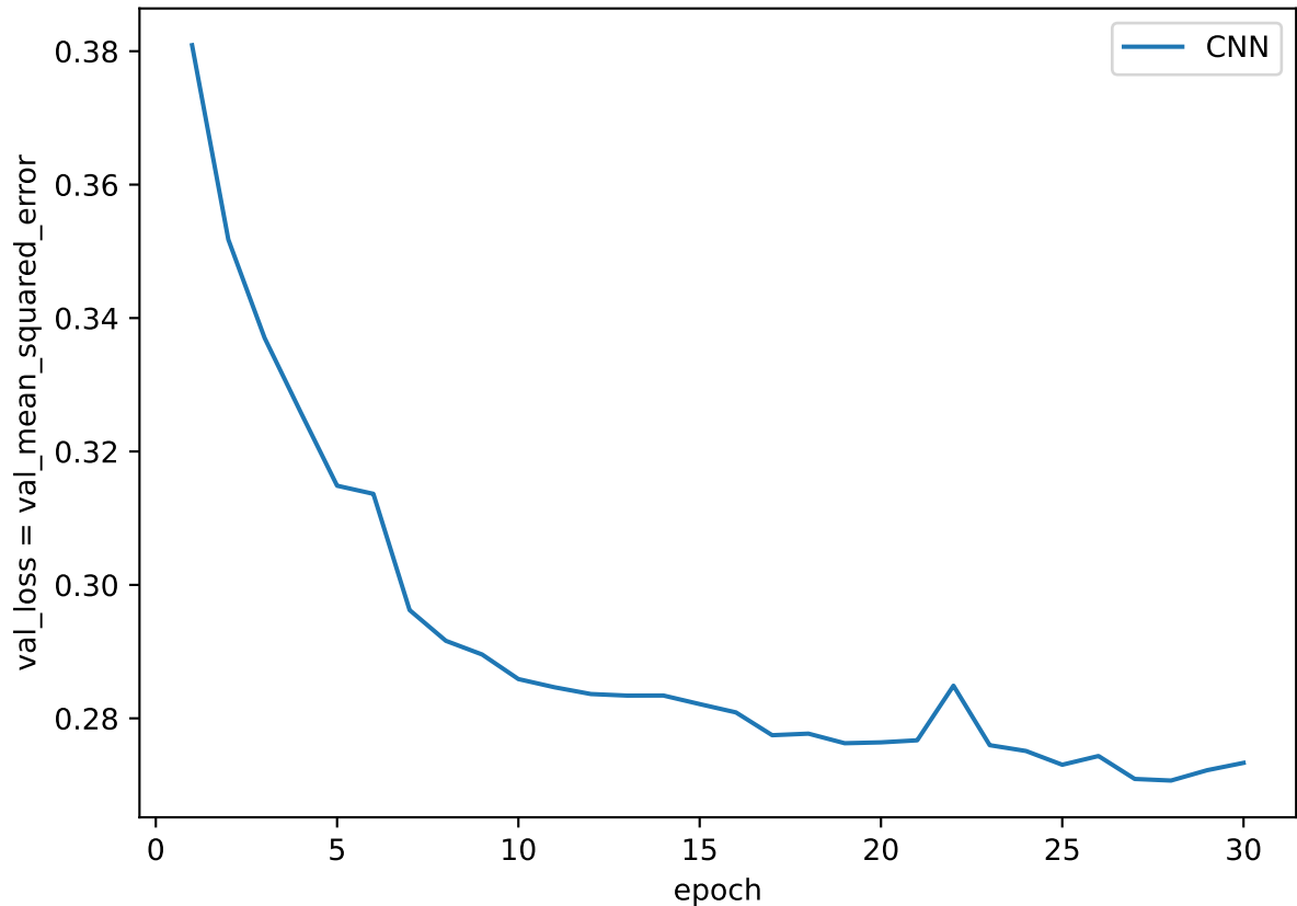
Potek učenja - Kernel 3x3
