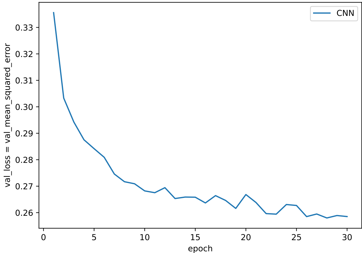
Potek učenja - Kernel (9x9)
