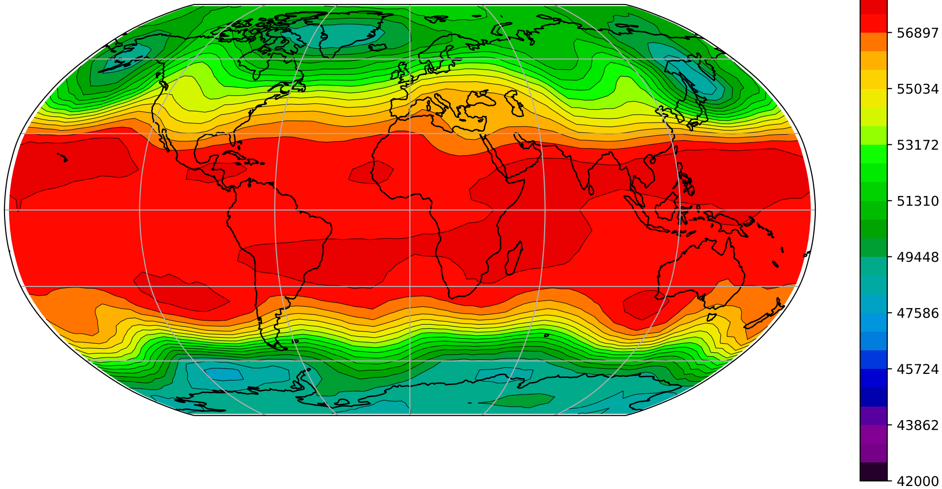
Z500, 2 dni od zacetnega dne 0
