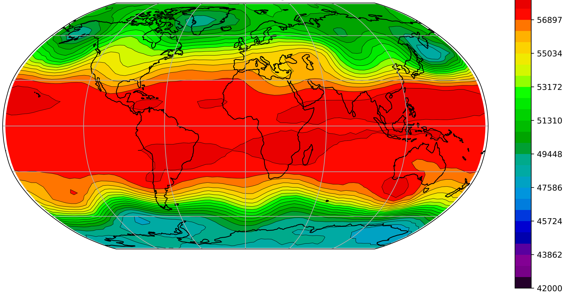
Z500, 4 dni od zacetnega dne 0
