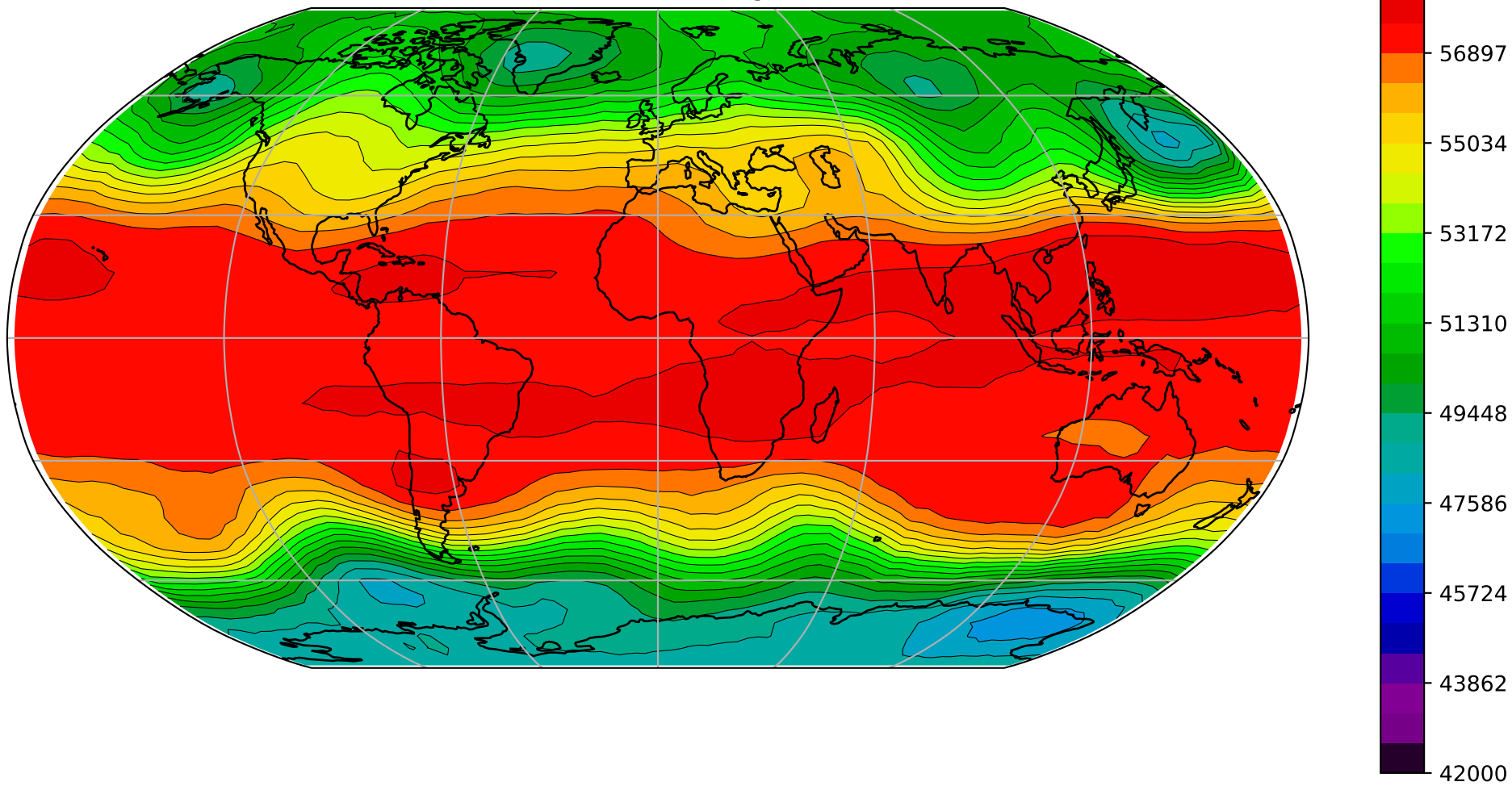
Z500, 5 dni od zacetnega dne 0
