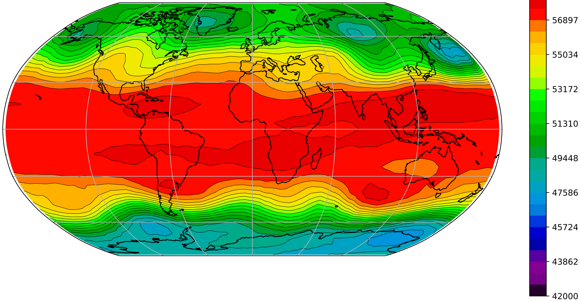
Z500, 6 dni od zacetnega dne 0
