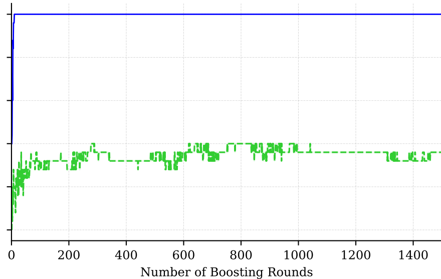
AdaBoost.M1 — ECG200
