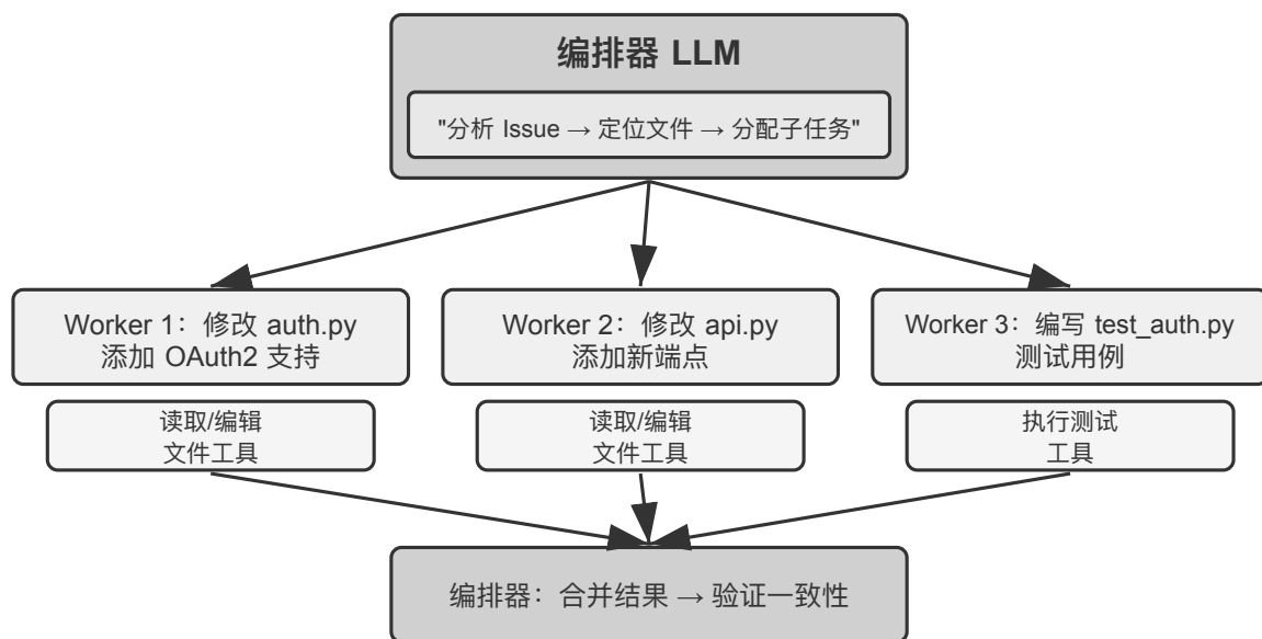
图 1-8 编排器-工作器模式：多文件代码修改
