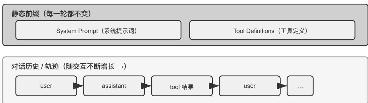
图 2-4 Agent 每次调用模型时的上下文构成
