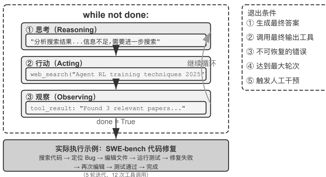
图 1-10 自主 Agent 的执行循环
