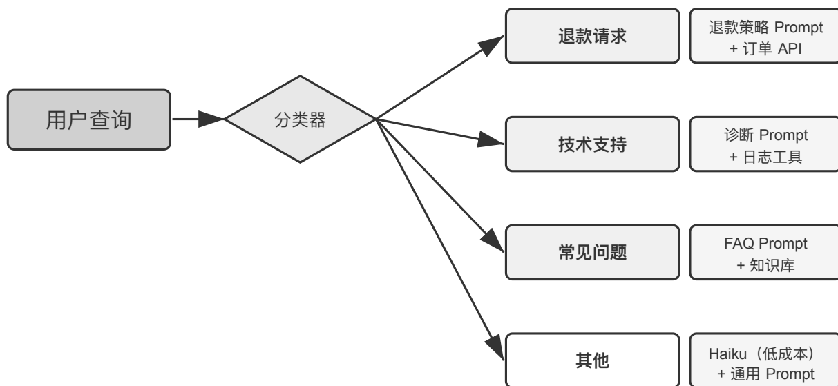
图 1-6 路由模式：客户服务分类
