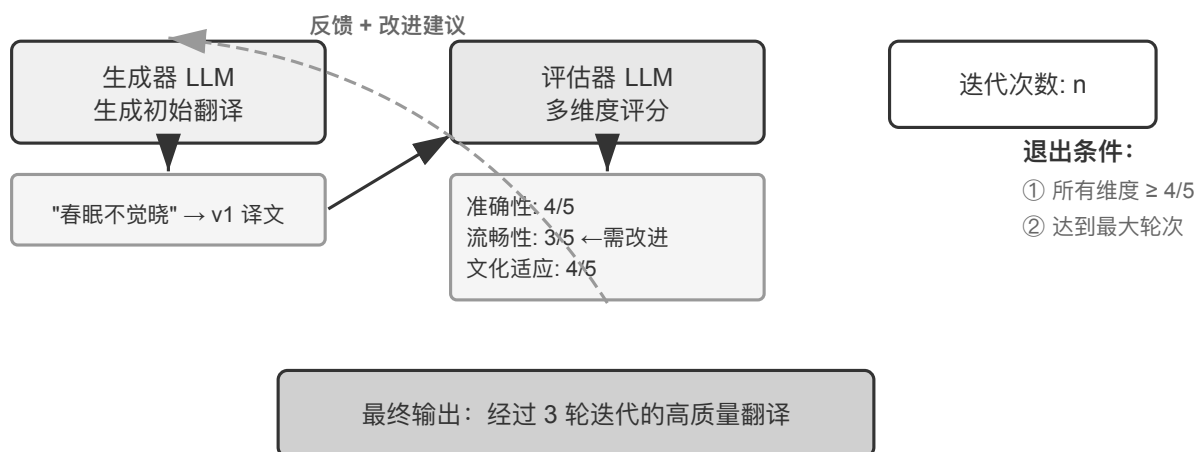
图 1-9 评估器-优化器模式：文学翻译迭代
