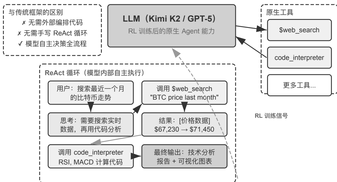
图 1-3 原生工具调用驱动的 ReAct 执行过程
