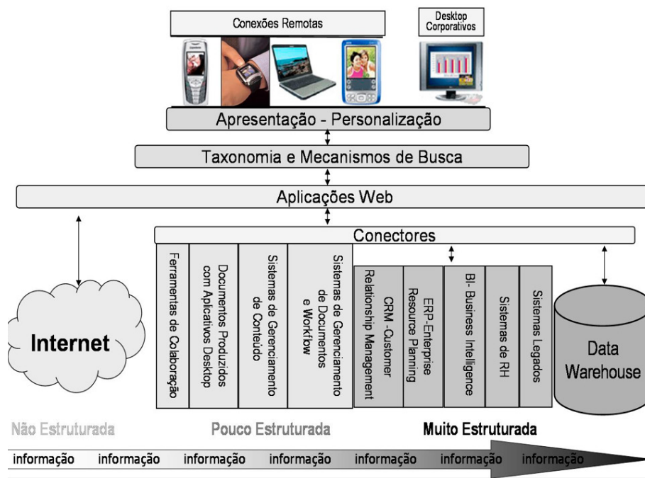
Figura – Componentes de um Portal Corporativo
