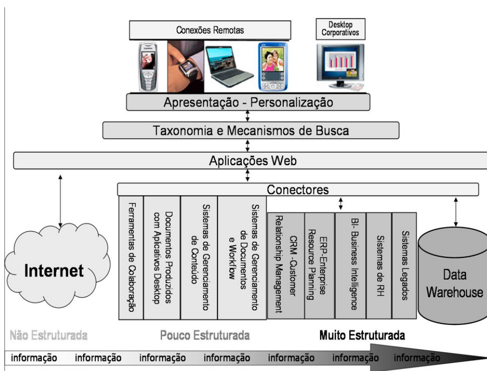
Figura – Arquitetura tecnológica de um portal corporativo
