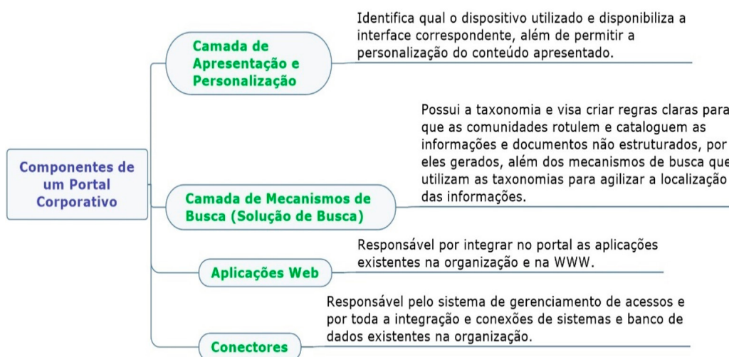
Figura – Componentes de um Portal Corporativo
