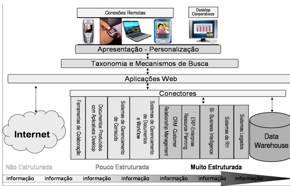
Figura – Arquitetura tecnológica de um portal corporativo.
