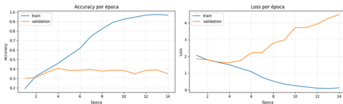
Figura 1. Evolución de accuracy y loss en el Experimento 1.
