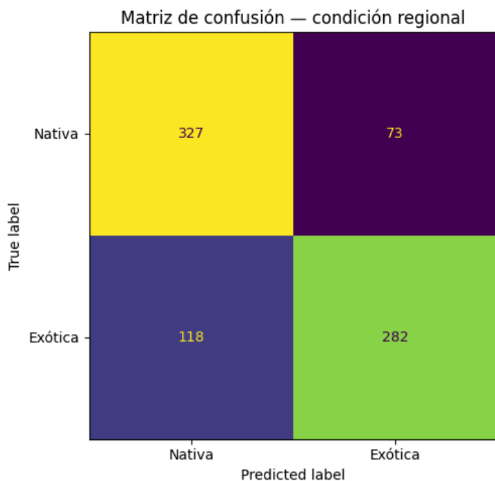
Figura 8. Matriz de confusión Nativa/Exótica - Experimento 2.
