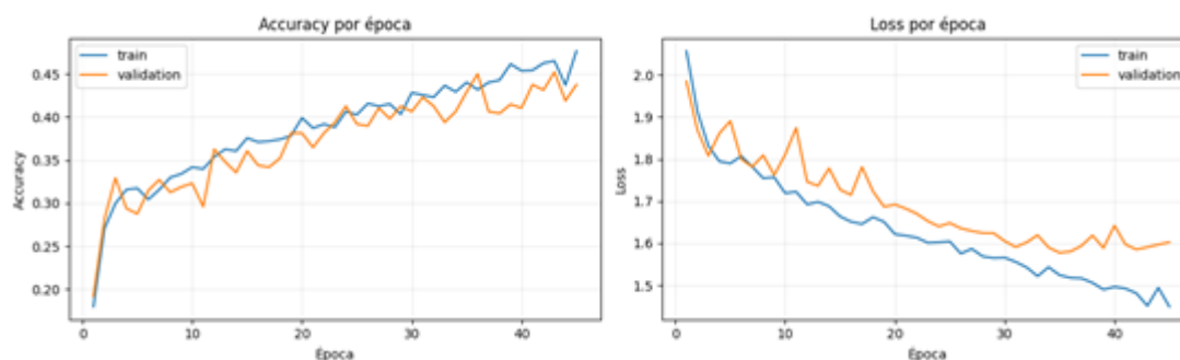
Figura 6. Evolución de accuracy y loss en el Experimento 3.
