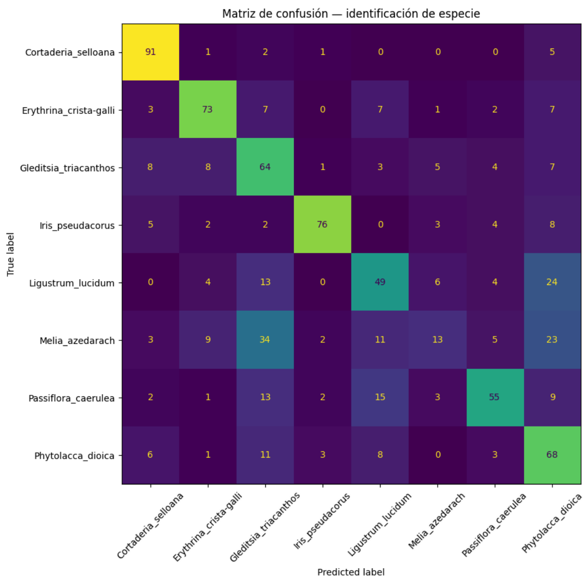
Figura 4. Matriz de confusión por especie - Experimento 2.
