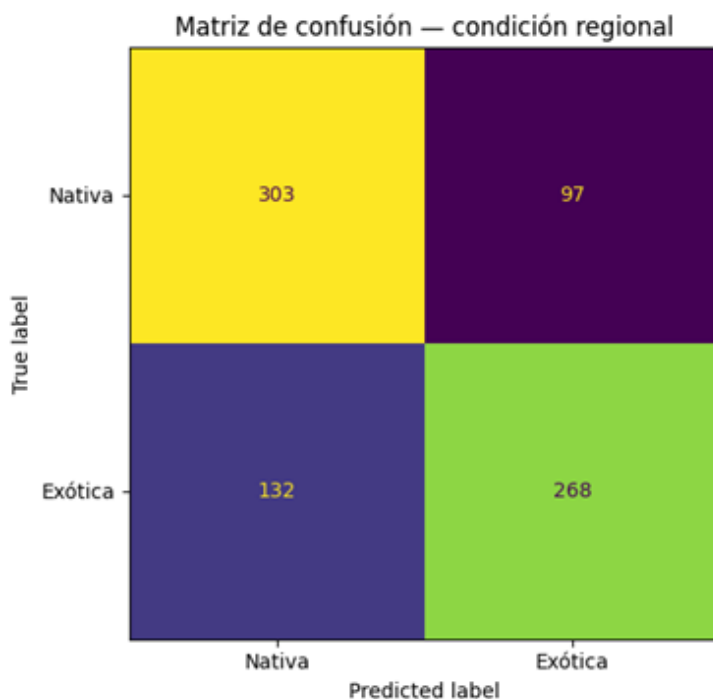
Figura 9. Matriz de confusión Nativa/Exótica - Experimento 3.
