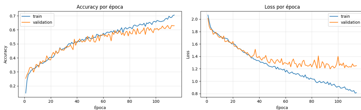
Figura 3. Evolución de accuracy y loss en el Experimento 2.
