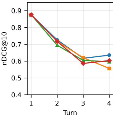
BGE-M3 (dense)
