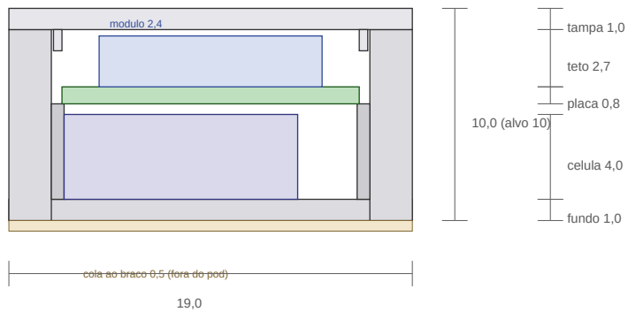
corte transversal (y, z), pelo meio da célula
