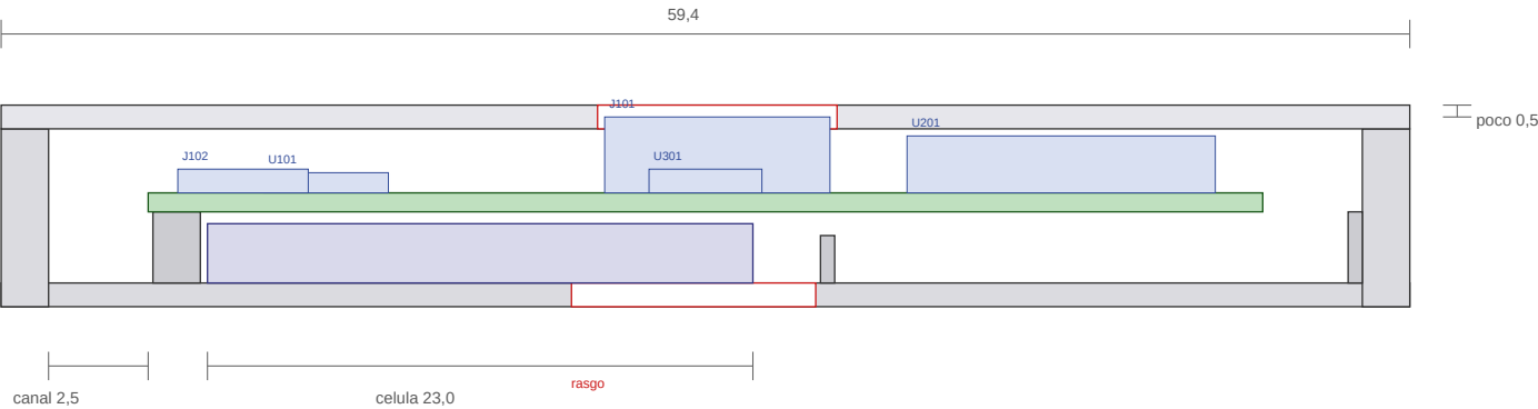
corte longitudinal (x, z), pelo eixo da placa; as pecas mais altas de cada bloco
