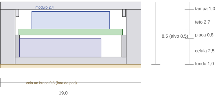
corte transversal (y, z), pelo meio da celula
