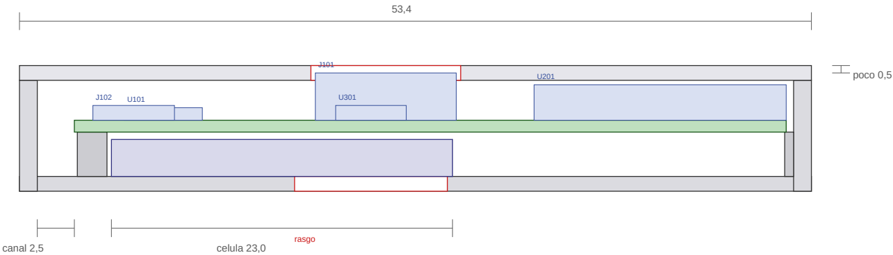
corte longitudinal (x, z), pelo eixo da placa; as pecas mais altas de cada bloco
