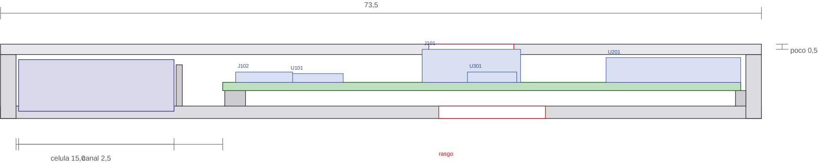
corte longitudinal (x, z), pelo eixo da placa; as pecas mais altas de cada bloco
