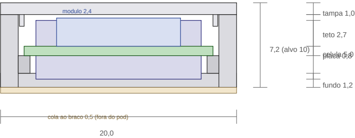
corte transversal (y, z), pelo meio da celula
