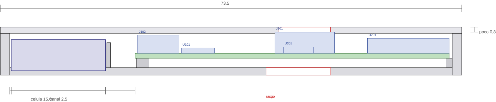
corte longitudinal (x, z), pelo eixo da placa; as pecas mais altas de cada bloco
