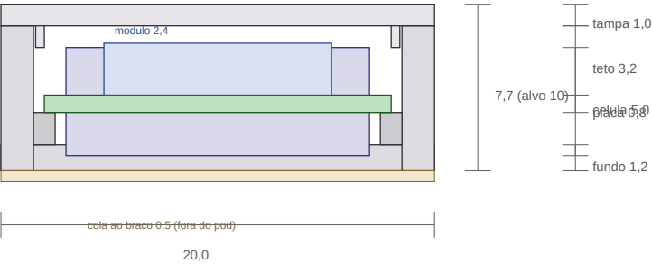
corte transversal (y, z), pelo meio da celula
