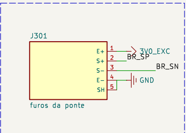
Ponte de extensometros
