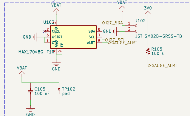
Medidor de carga e celula
