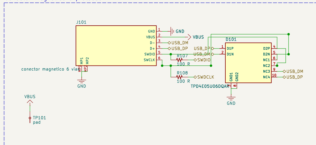
Conector magnetico e protecao
