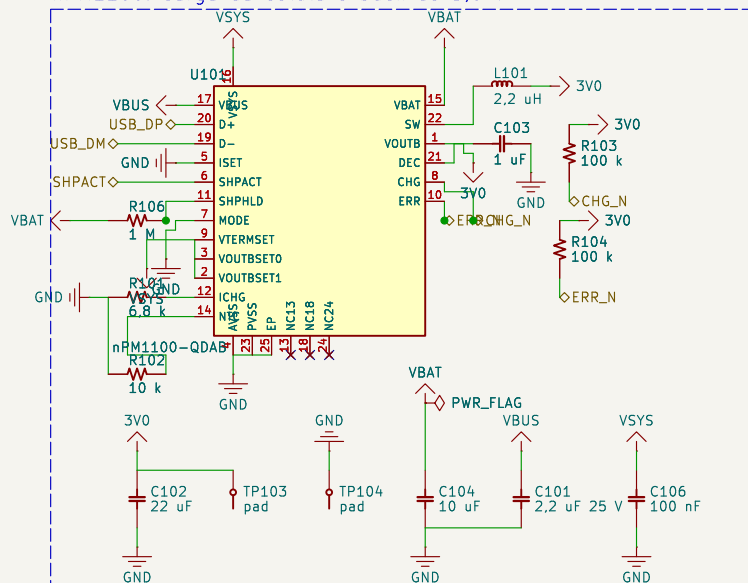
nPM1100: carga da celula e buck de 3,0 V
