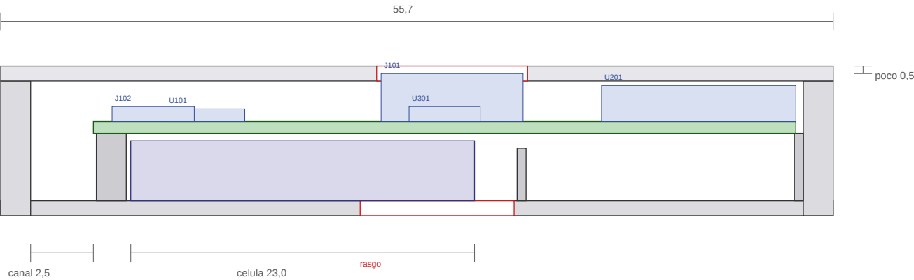
corte longitudinal (x, z), pelo eixo da placa; as pecas mais altas de cada bloco
