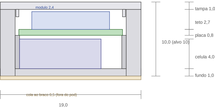
corte transversal (y, z), pelo meio da celula
