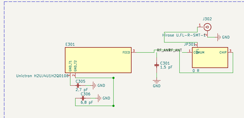
Antena de chip e rede pi
