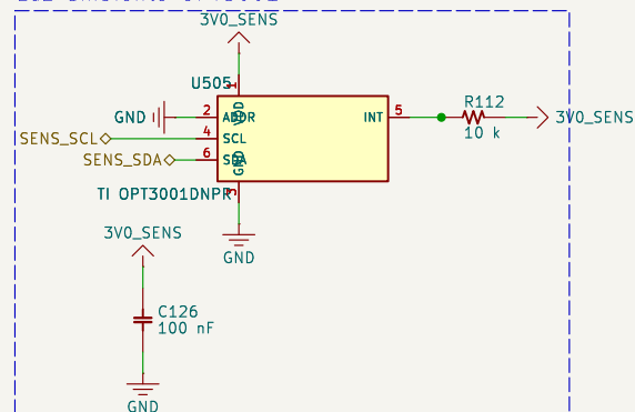
Luz ambiente OPT3001
