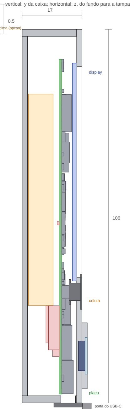
Corte A-A pelo comprimento
