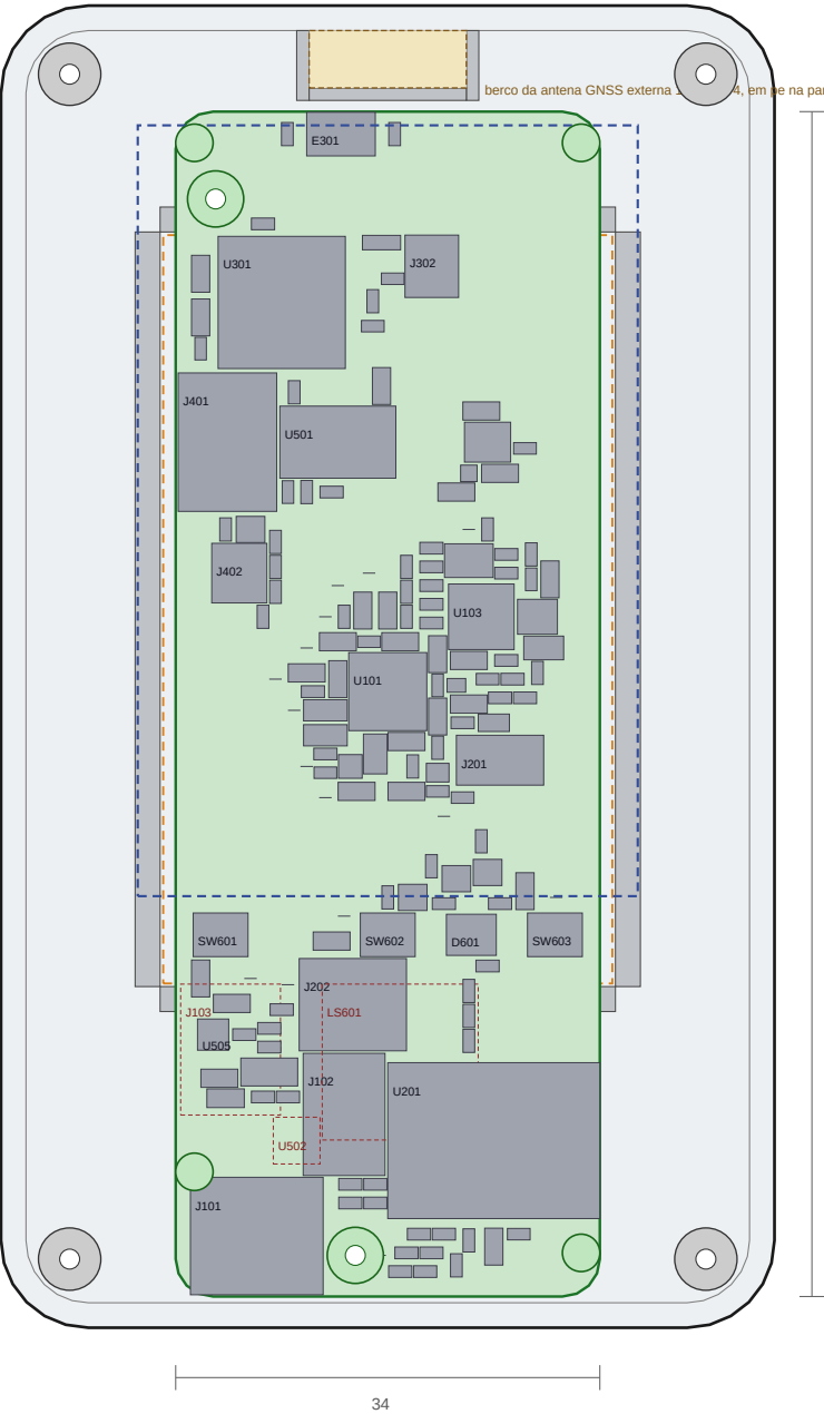
Por dentro: concha, placa, celula (tracejada) e display (tracejado)
