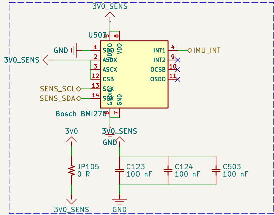
IMU BMI270
