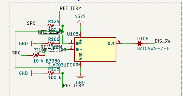
Corte termico da carga solar
