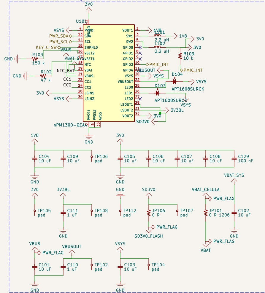
nPM1300: entrada, carga e os dois bucks
