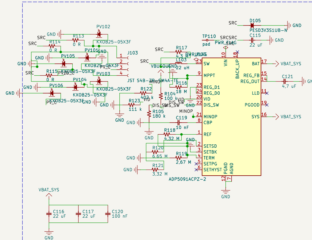
Colheita solar ADP5091
