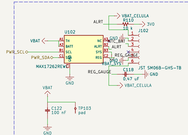
Medidor de bateria e celula
