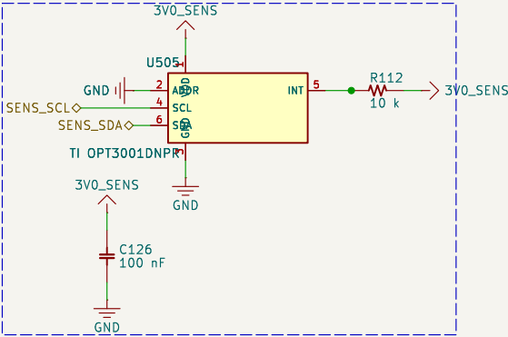
Luz ambiente OPT3001
