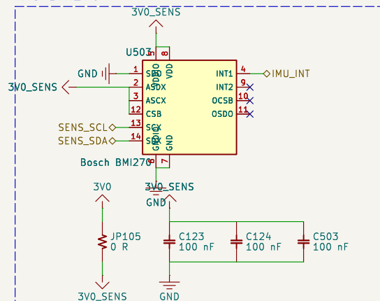
IMU BMI270
