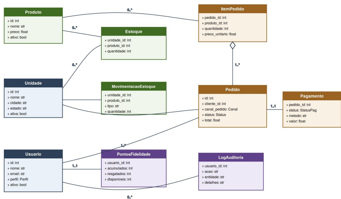
Figura 3 — Diagrama de Classes (visão de domínio)
