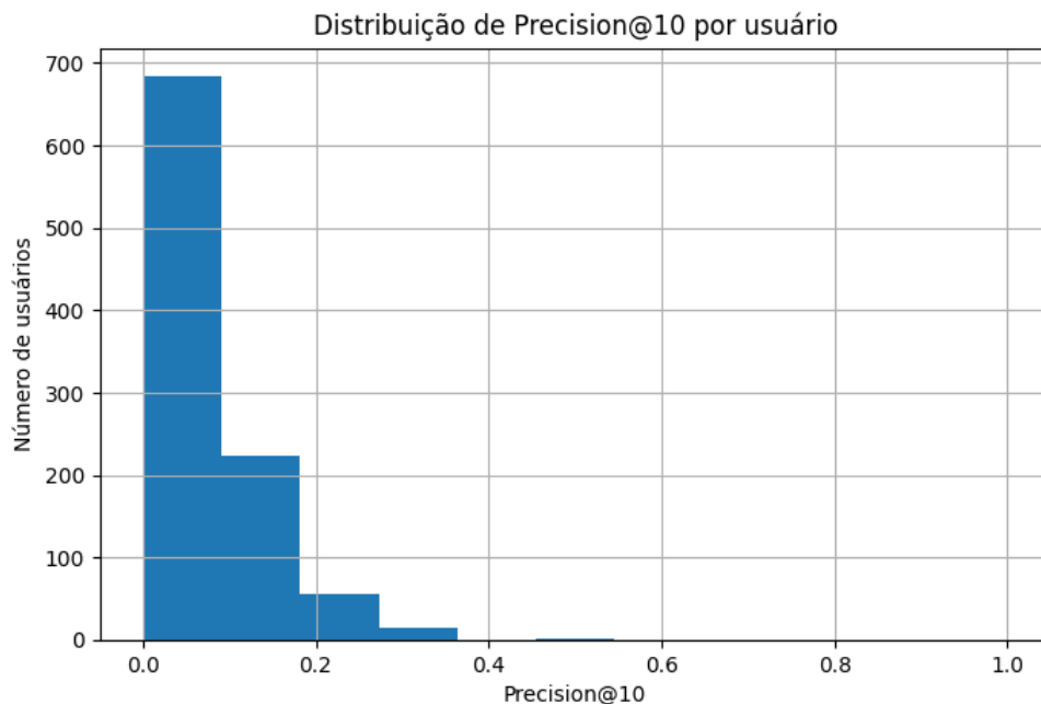
Figura 5: Distribuição da Precisão@10 entre usuários avaliados.
