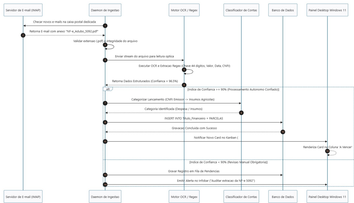
Figura 5: Diagrama de Sequência — Ingestão e Processamento Autônomo de PDF
