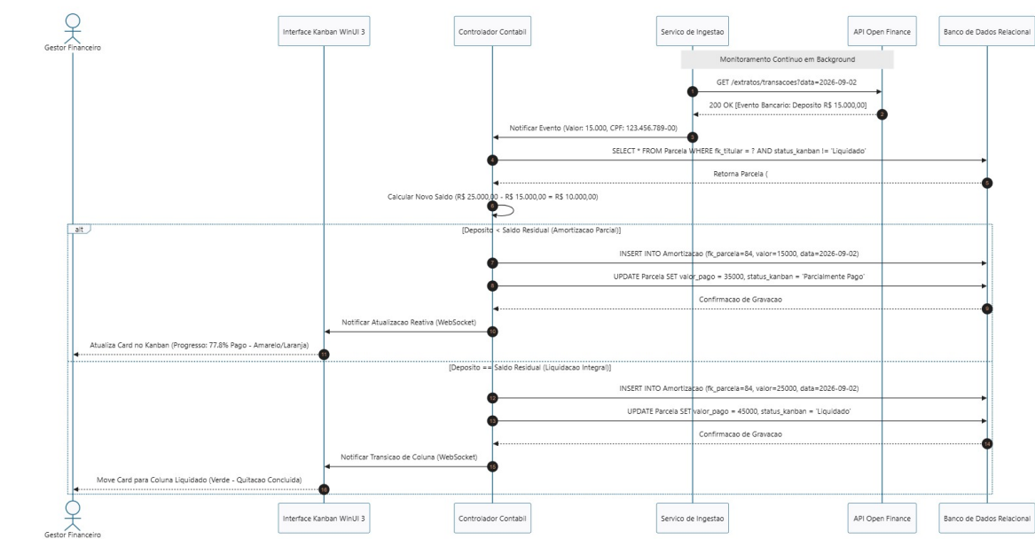
Figura 4: Diagrama de Sequência — Baixa de Amortização via Open Finance
