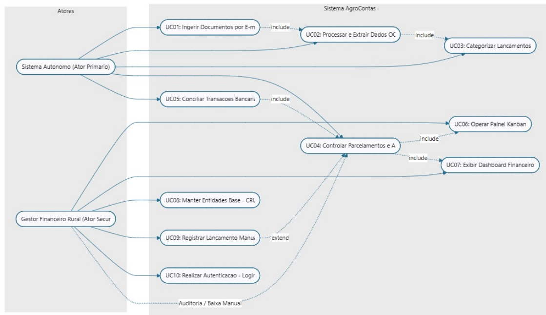
Figura 2: Diagrama de Caso de Uso — AgroContas
