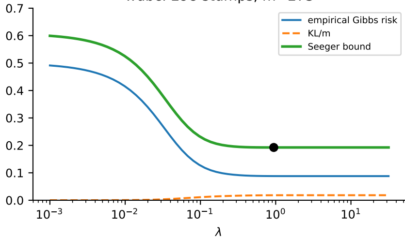
wdbc: 298 stumps, m=273
