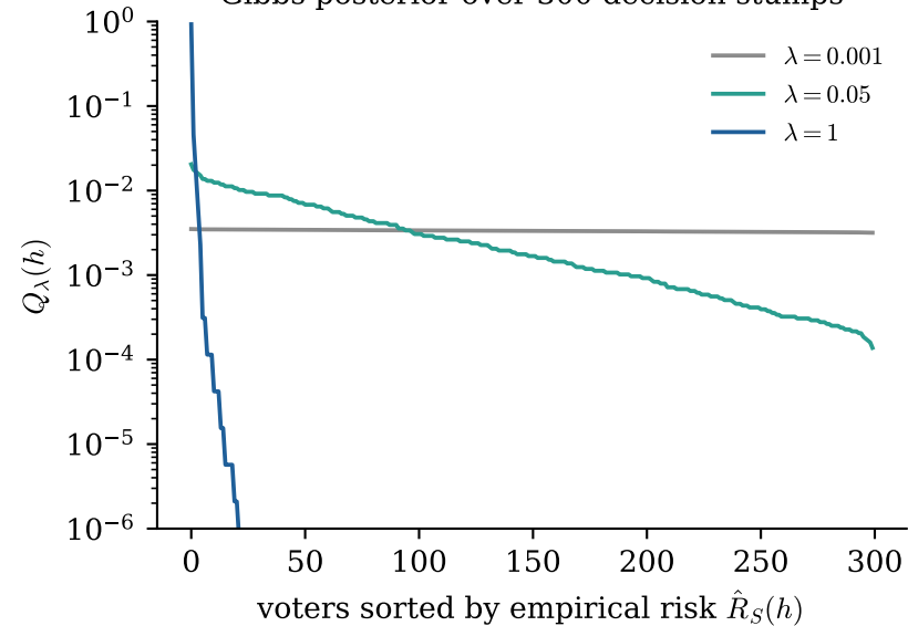
Gibbs posterior over 300 decision stumps
