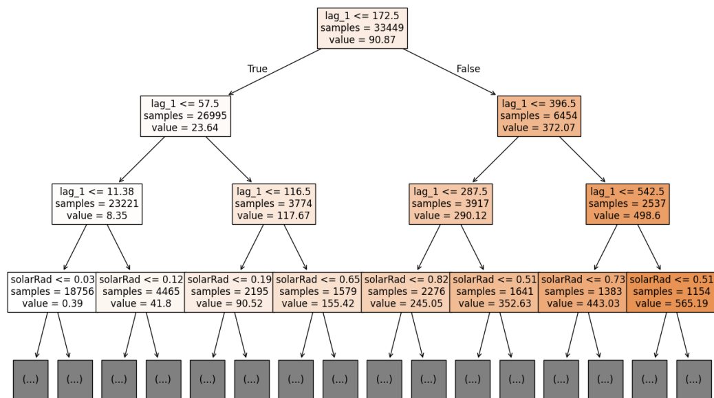
Ilustración 10 – SimpleTree
