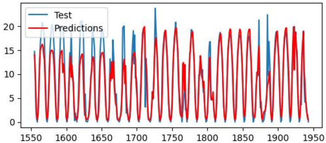
Ilustración 18 - Predicciones (Lorca)
