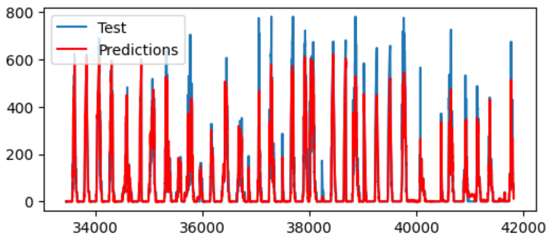
Ilustración 17 - Predicciones (CTC)
