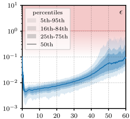
kinematic parameters
