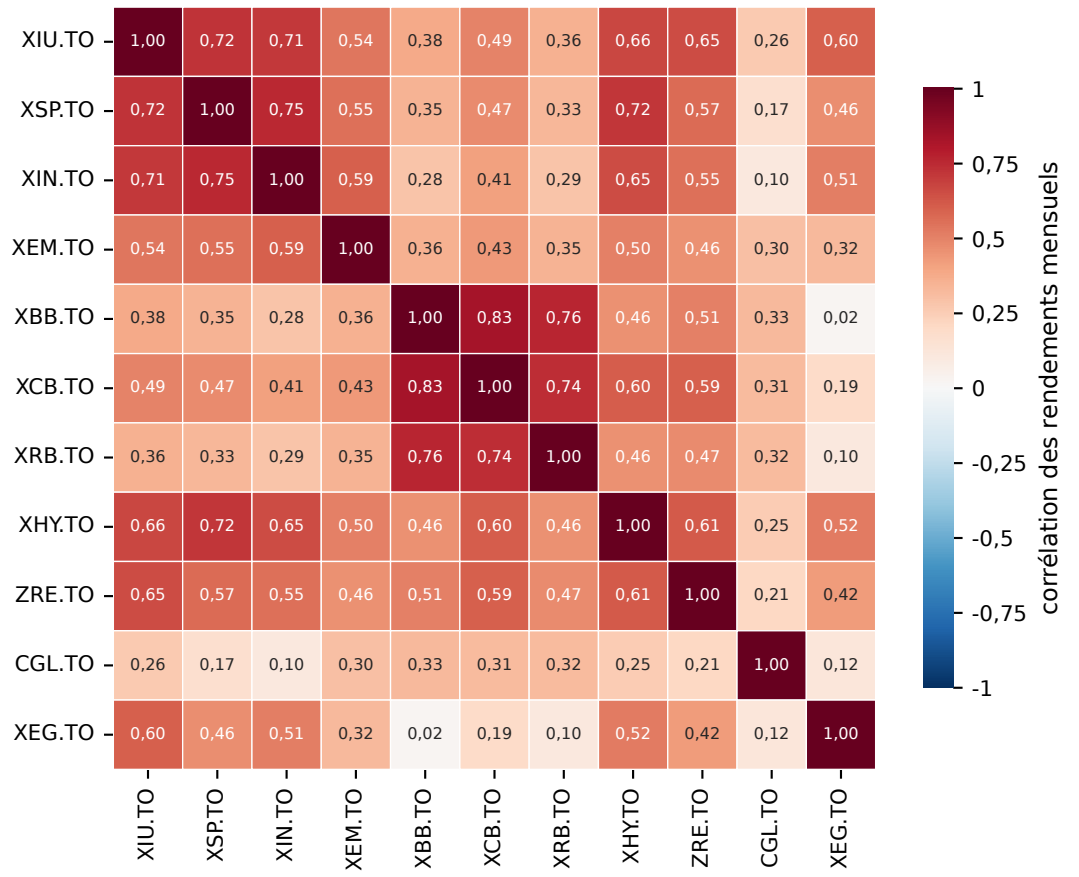
Corrélations, FNB canadiens multi-actifs (CAD), 2011-01 à 2026-07, estimateur Ledoit-Wolf
