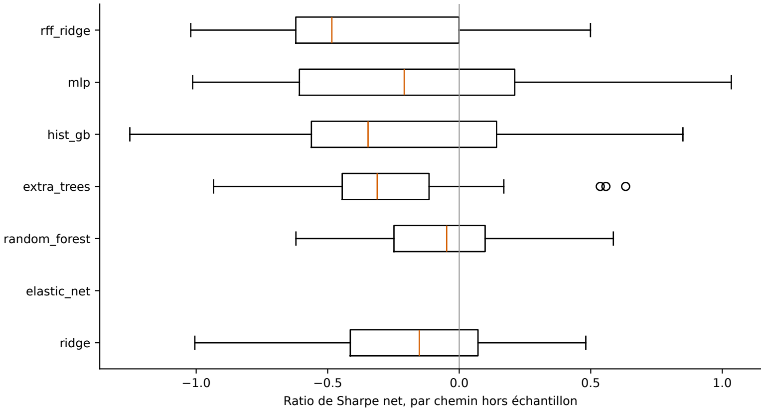
Canada (50 titres TSX) : Sharpe net sur les 28 chemins CPCV (purge et embargo)
