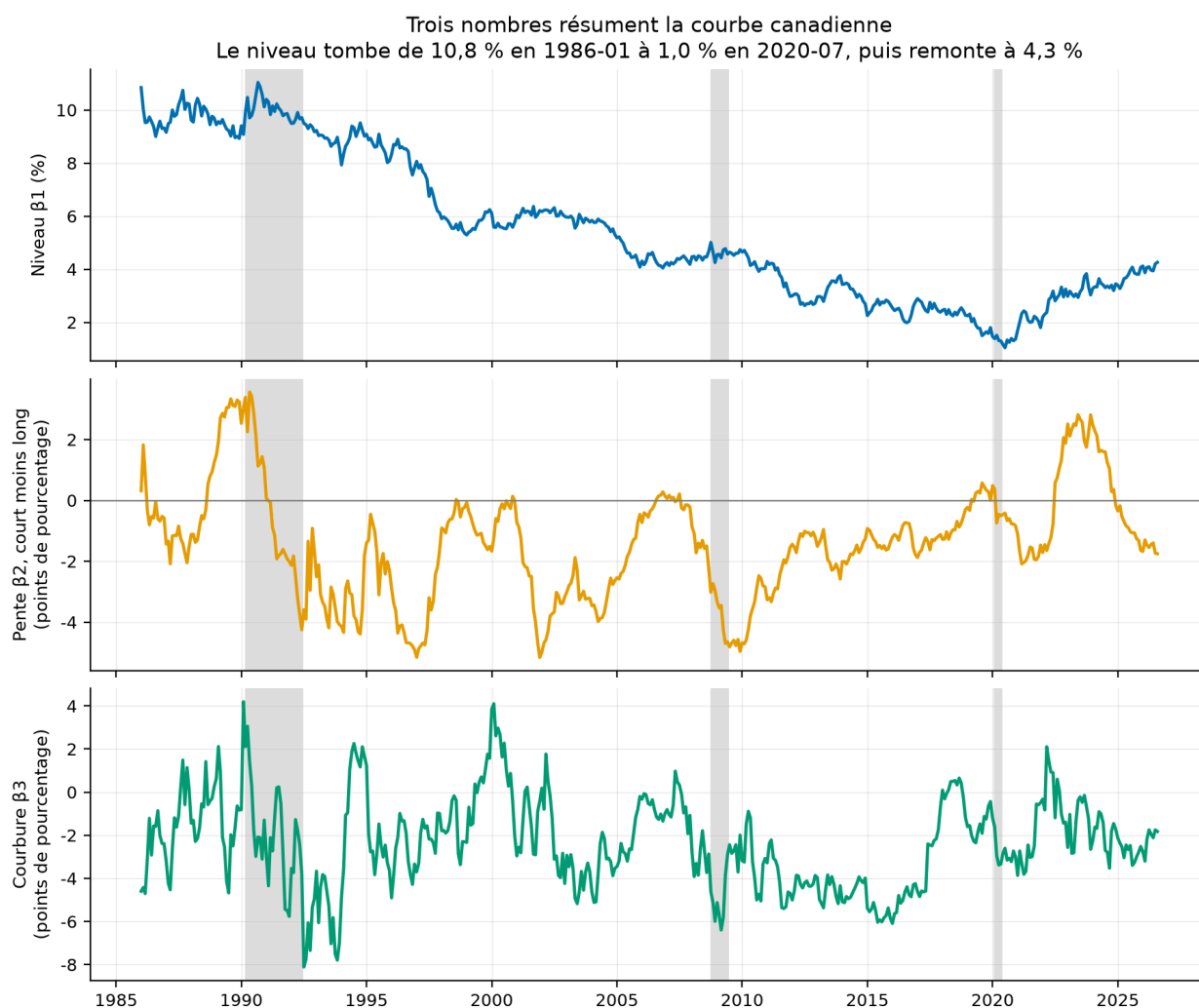
Fig. 1. – Facteurs Nelson-Siegel
