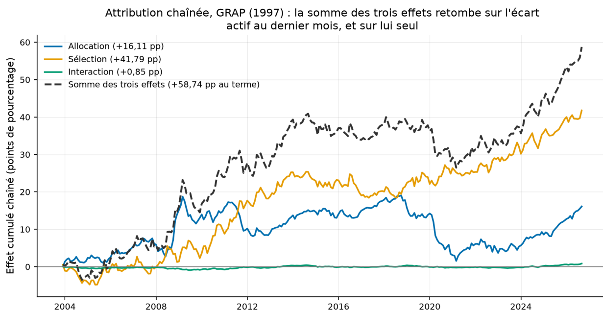
Fig. 3. – Attribution chaînée
