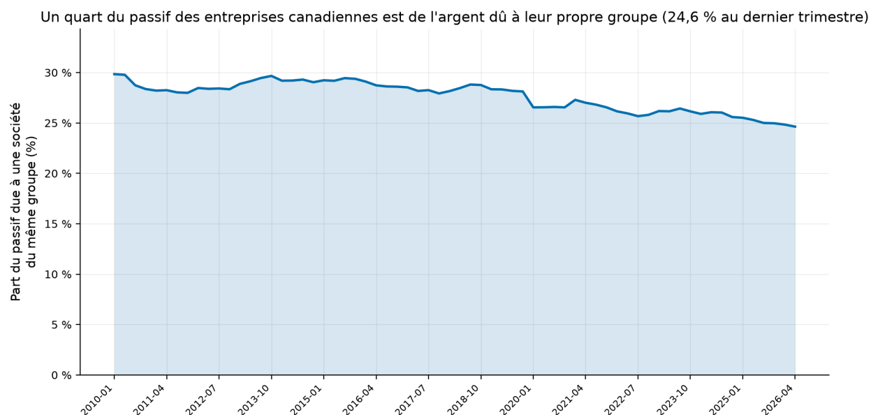
Fig. 4. – La part du passif due au groupe, trimestre par trimestre
