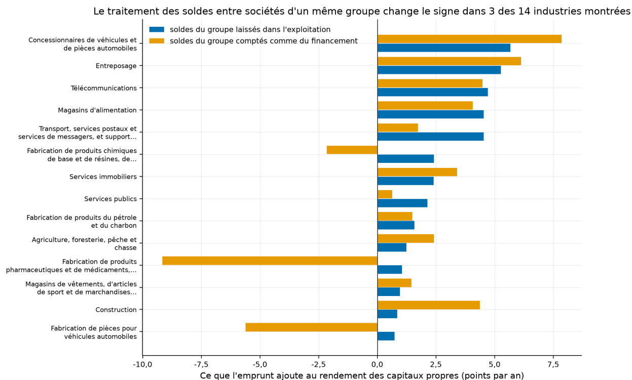
Fig. 3. – La même industrie lue deux fois
