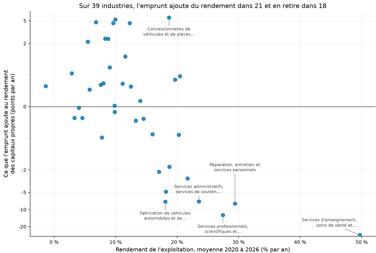
Fig. 2. – Chaque industrie, son affaire et ce que l'emprunt y ajoute
