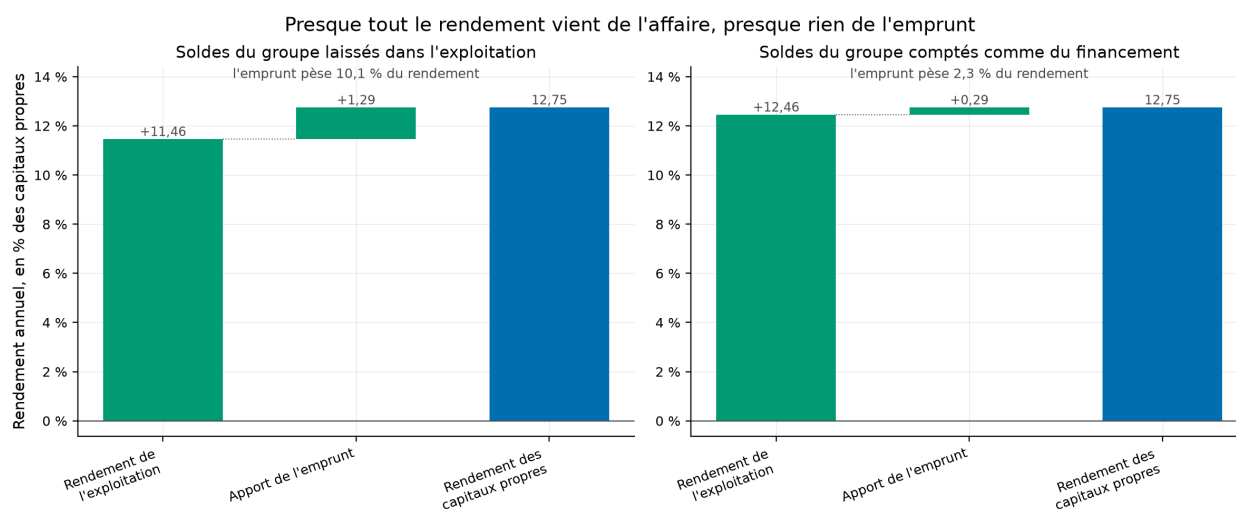
Fig. 1. – La décomposition du rendement, dans les deux lectures
