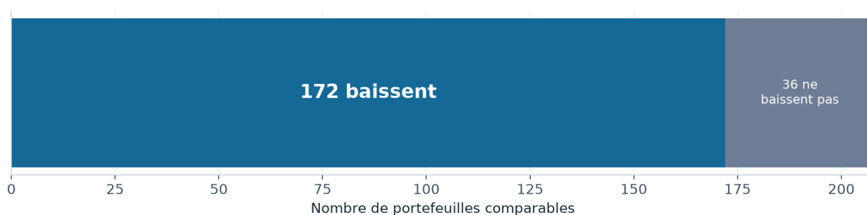
Fig. 1. – Nombre de portefeuilles dont le rendement baisse après publication
