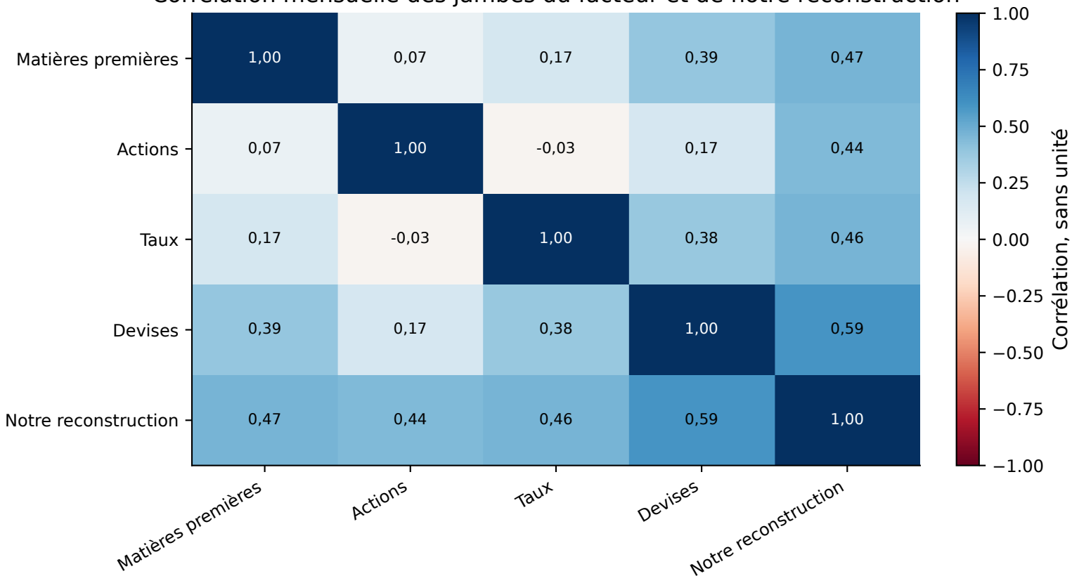
Corrélation mensuelle des jambes du facteur et de notre reconstruction
