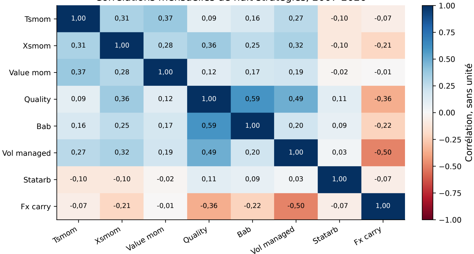
Corrélations mensuelles de huit stratégies, 2007-2026
