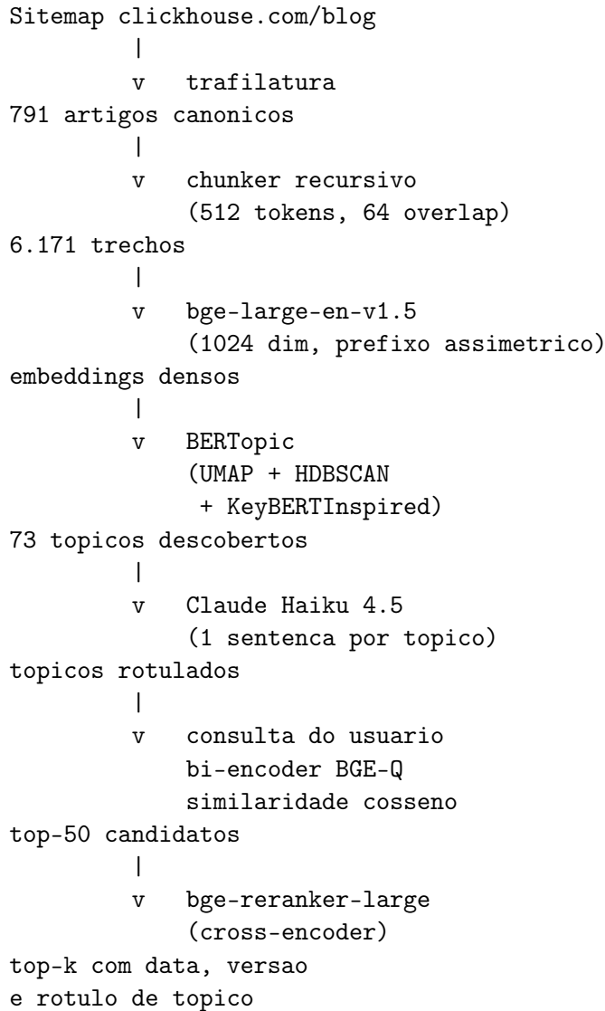
Figura 1: Arquitetura do pipeline de recuperação densa proposto.
