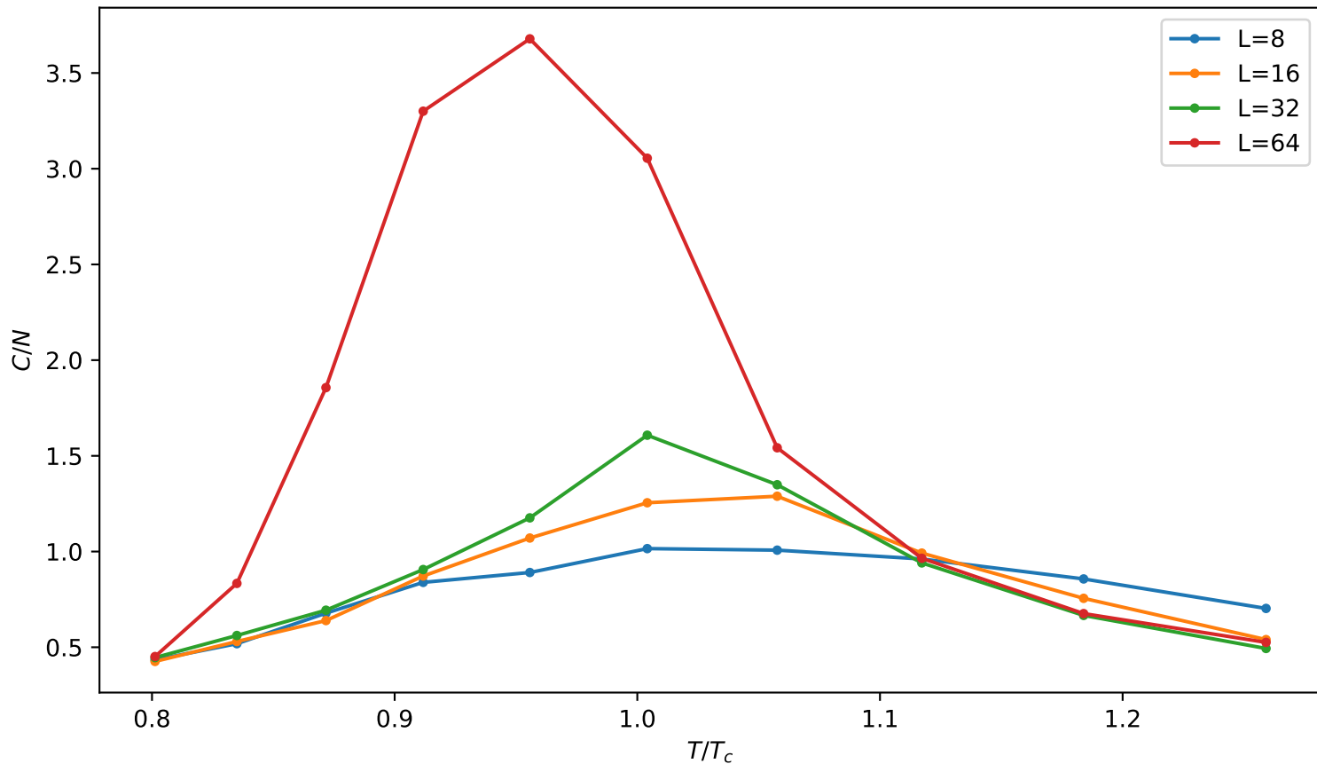
Specific heat per spin - wolff
