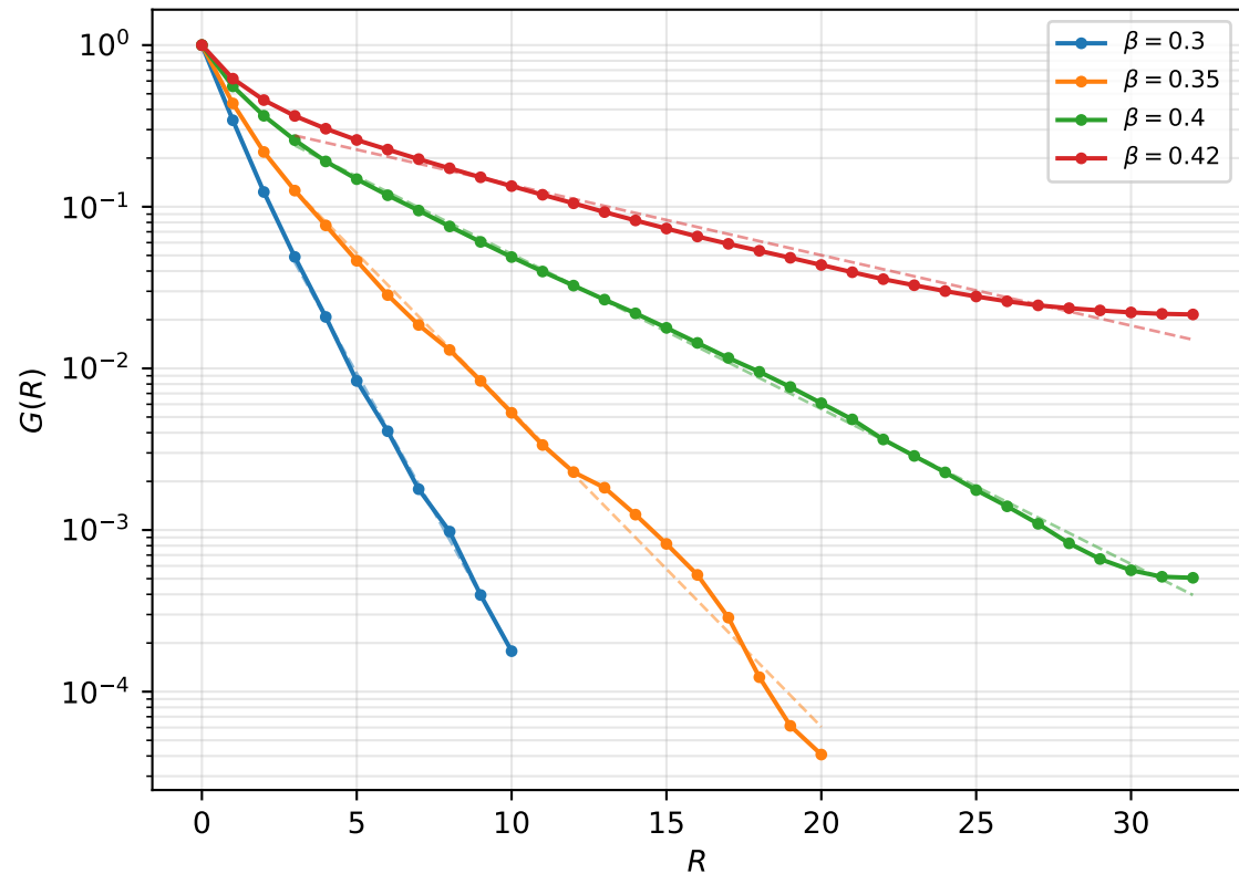
Cluster estimator
