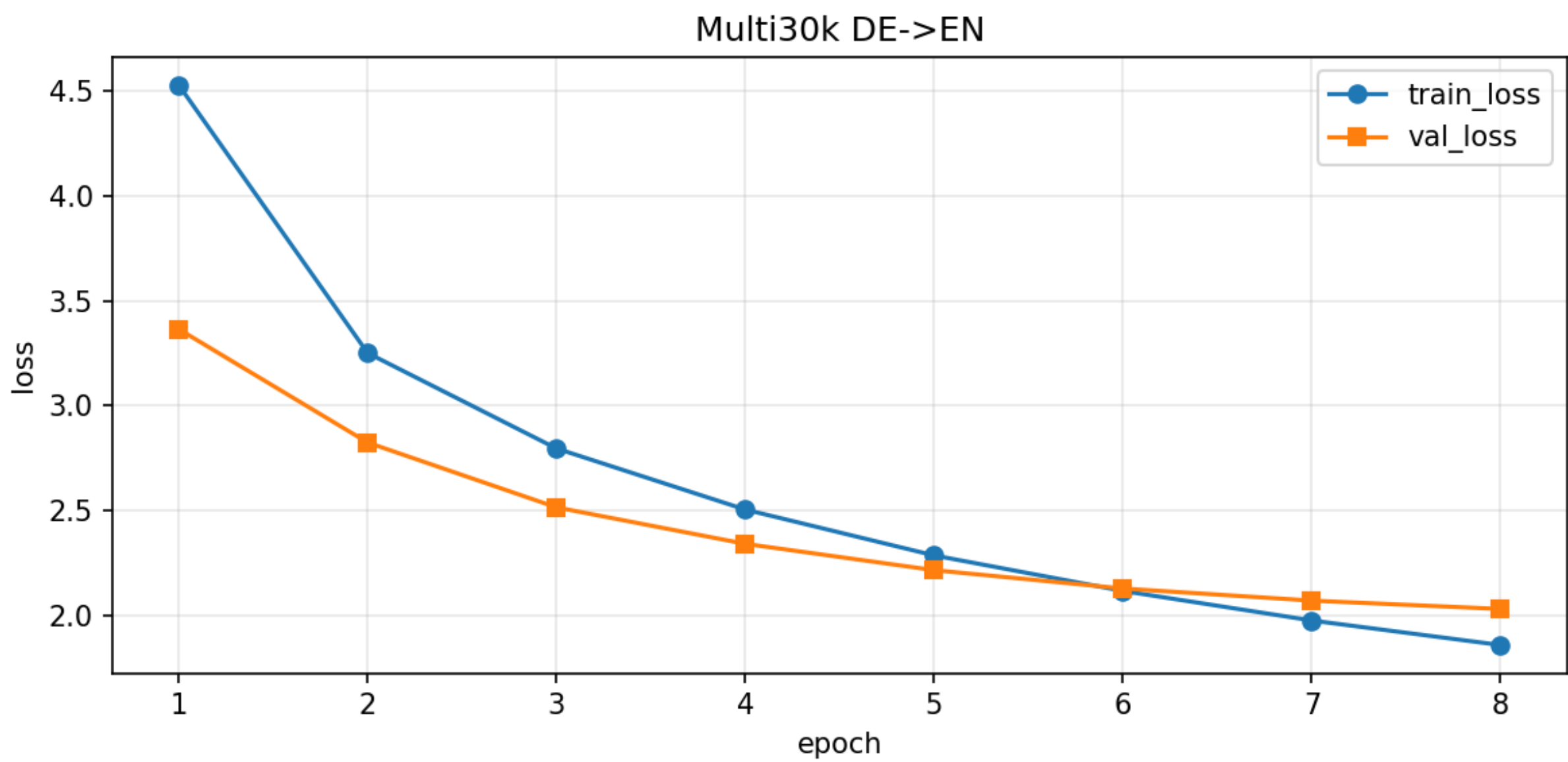
翻译任务 Loss 曲线
