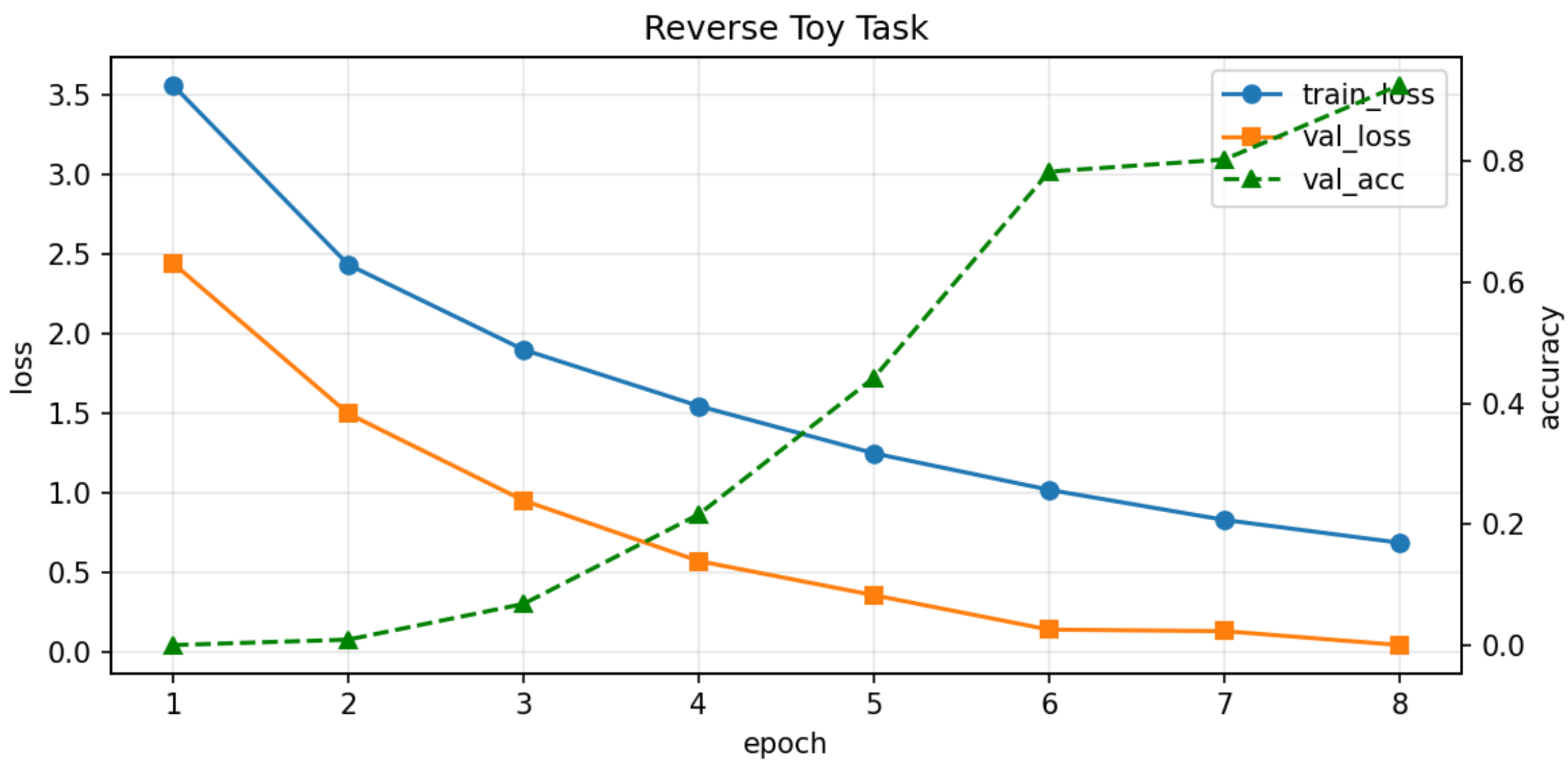
序列反转任务 Loss 曲线
