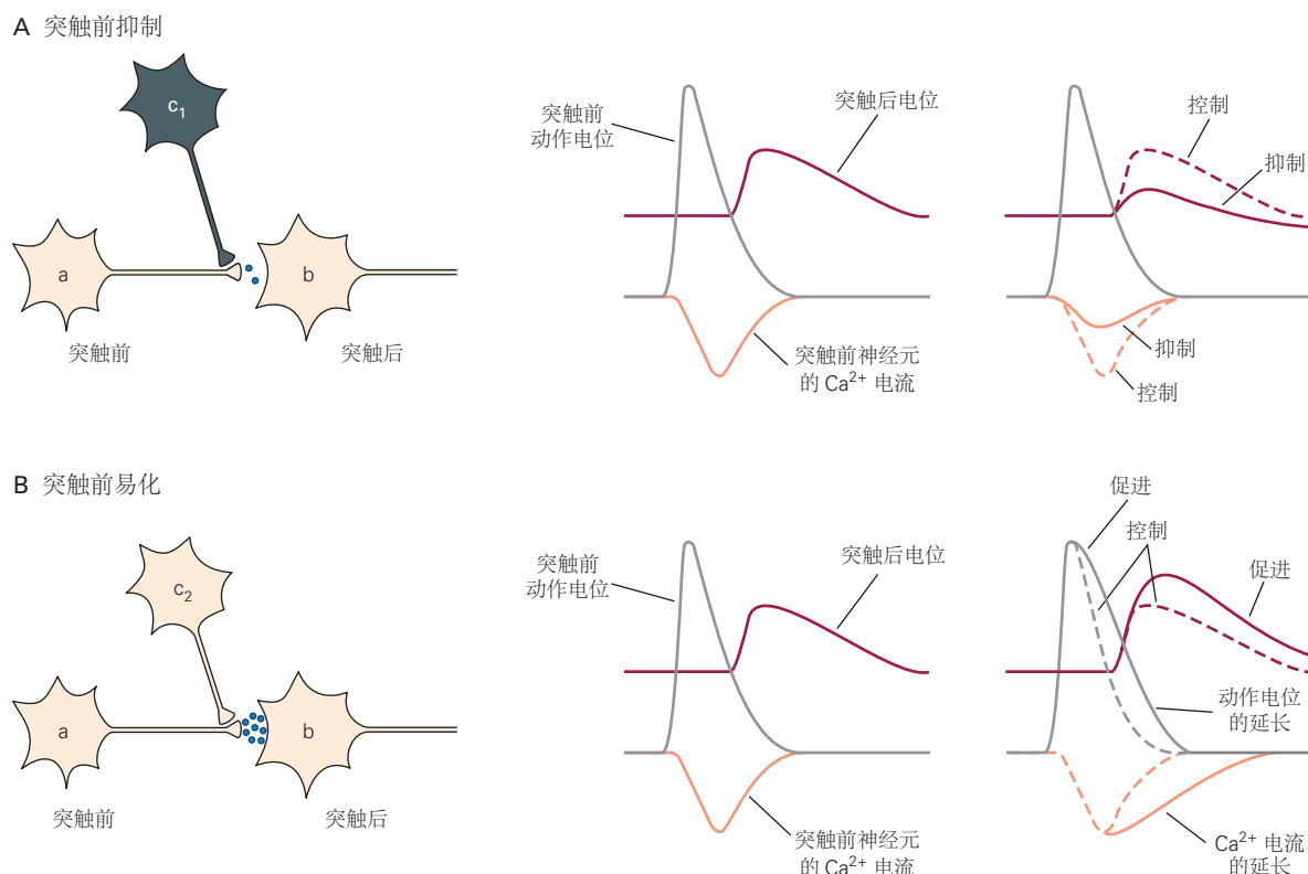
图 15.6.1: 轴-轴突触可以抑制或促进突触前细胞释放递质。A. 抑制性神经元 ( c_1 ) 在神经元 a 的轴突末梢形成突触。细胞 c_1 释放递质会激活末梢代谢受体，从而抑制末梢 \text{Ca}^{2+} 电流，减少了细胞 a 释放到细胞 b 的递质数量。细胞 a 递质释放的减少反过来又降低了细胞 b 中兴奋性突触后电位的幅度，这一过程称为突触前抑制。B. 促进性神经元 ( c_2 ) 在神经元 a 的轴突末梢形成突触。细胞 c_2 释放递质会激活末梢的促代谢受体，从而降低末梢的 \text{K}^+ 电流，从而延长动作电位并增加 \text{Ca}^{2+} 流入细胞 a 。这增加了从细胞 a 到细胞 b 的递质释放，从而增加了细胞 b 中兴奋性突触后电位的大小，这一过程称为突触前促进。
