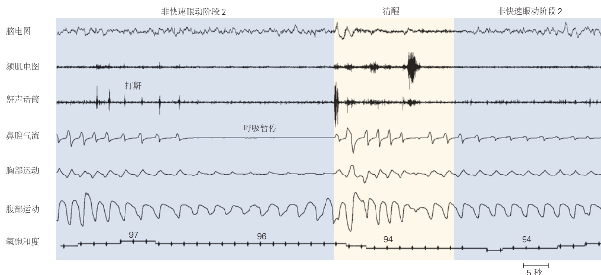
图 44.5.1: 睡眠呼吸暂停发作。在这个多导睡眠图的开始，一个人处于非快速眼动阶段 2 睡眠。检测到一些打鼾，但鼻腔气流良好且氧饱和度正常。然后，个体会出现阻塞性呼吸暂停，没有鼻腔气流；然而，呼吸努力仍然存在（由腹部运动显示）。呼吸暂停由短暂的觉醒（低电压快速脑电图）终止，伴随着响亮的鼾声、肌电图活动增加、呼吸努力增强和气道开放。氧饱和度下降约 3%，在呼吸暂停结束约 15 秒后达到最低点，因为血液从肺部流到测量氧饱和度的指尖需要时间。
