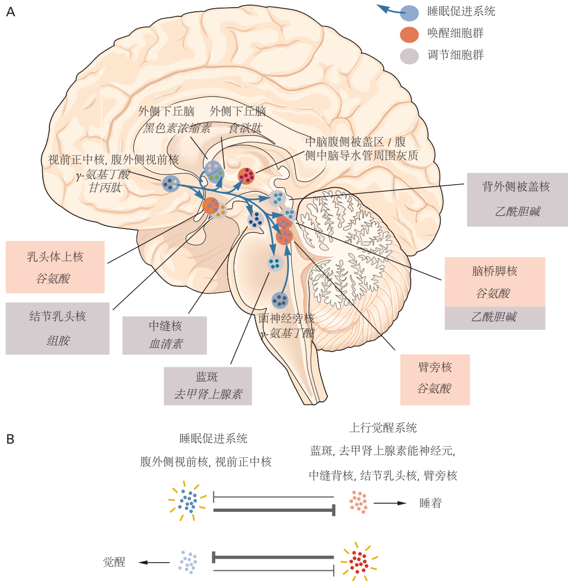
图 44.2.2: 促进睡眠的通路。A. 如图 44.2.1 所示，上行觉醒系统的组成部分从促进睡眠的神经元接收抑制性的、主要是 \gamma -氨基丁酸能的输入。腹外侧视前核和视前正中核中的神经元支配整个觉醒促进系统，而面神经旁核中的神经元主要支配臂旁区域。许多腹外侧视前核神经元还含有甘丙肽（一种抑制肽）。如图 44.2.3 所示，外侧下丘脑中释放黑色素浓缩素的神经元可通过抑制附近的食欲能神经元以及导水管周围灰质中阻止快速眼动睡眠的神经元来促进快速眼动睡眠。B. 腹外侧视前核和正中视前核与上行觉醒系统相互抑制成分的触发器开关关系。当被激活时，促进睡眠的神经元会抑制上行觉醒系统的组成部分。然而，促进睡眠的细胞群也受到觉醒系统的抑制。最终效果是个人大部分时间都处于完全觉醒或睡眠状态，同时最大限度地减少过渡状态的时间。
